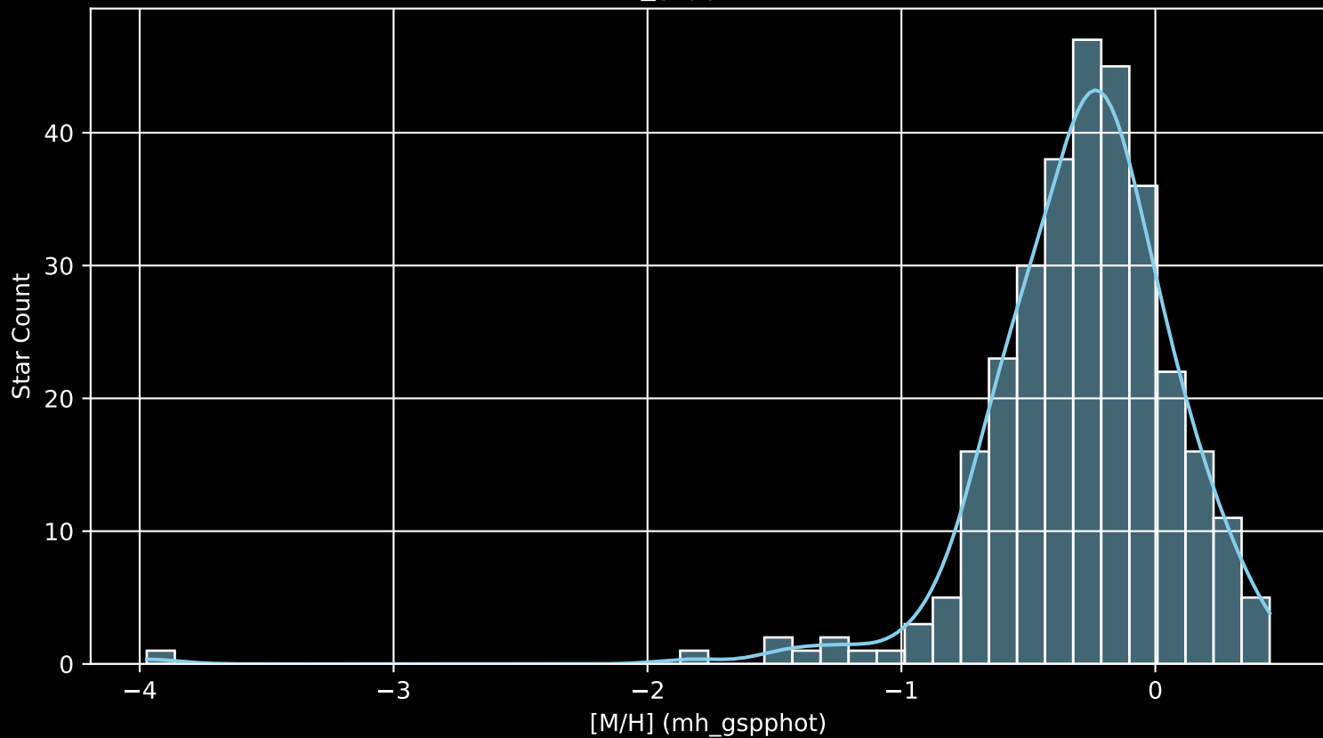
GALAH DR4 Field: [6965] [M/H] (mh_gspphot) (n= 306)
