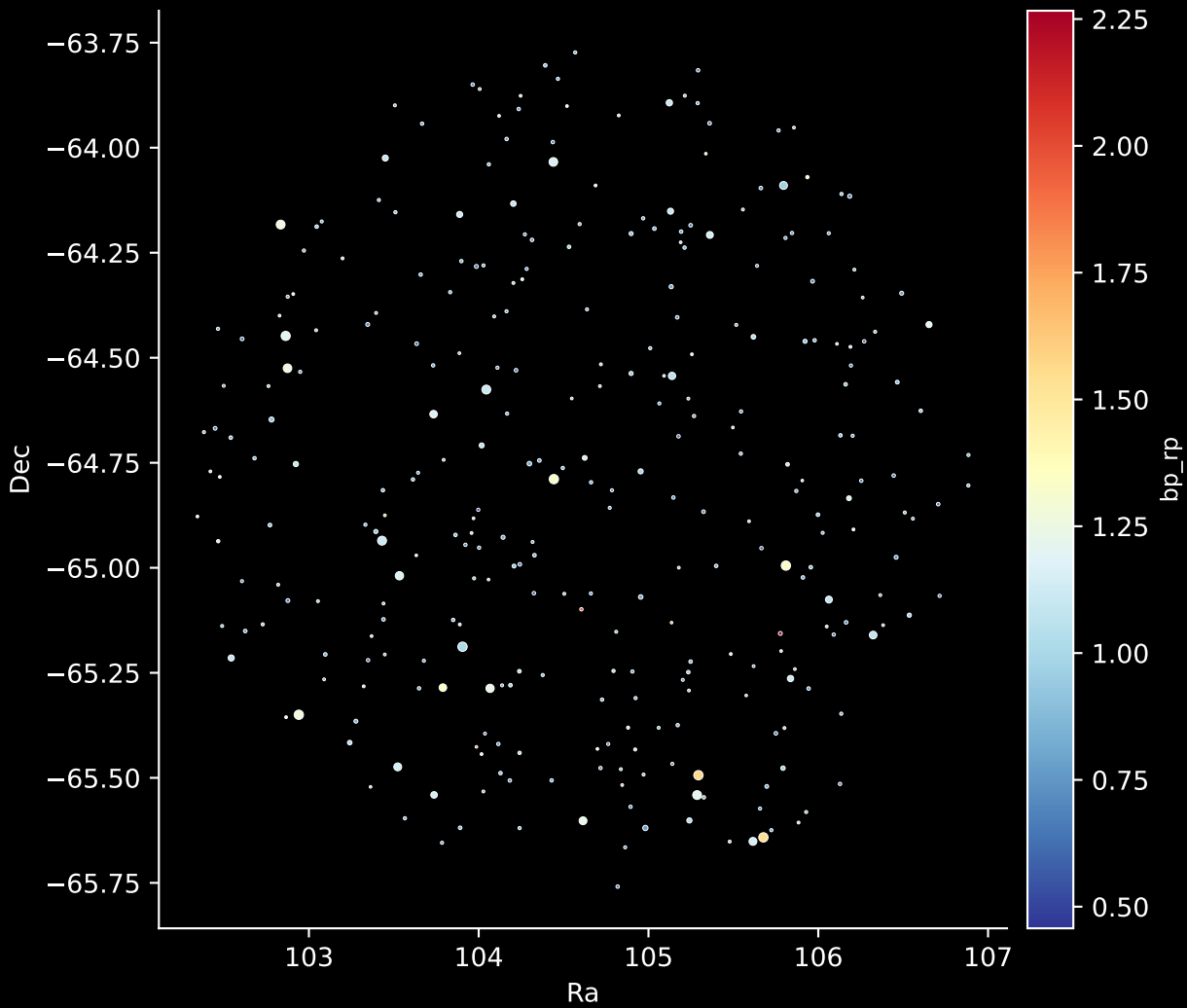
GALAH DR4 Field: [6965] Stars: 306
