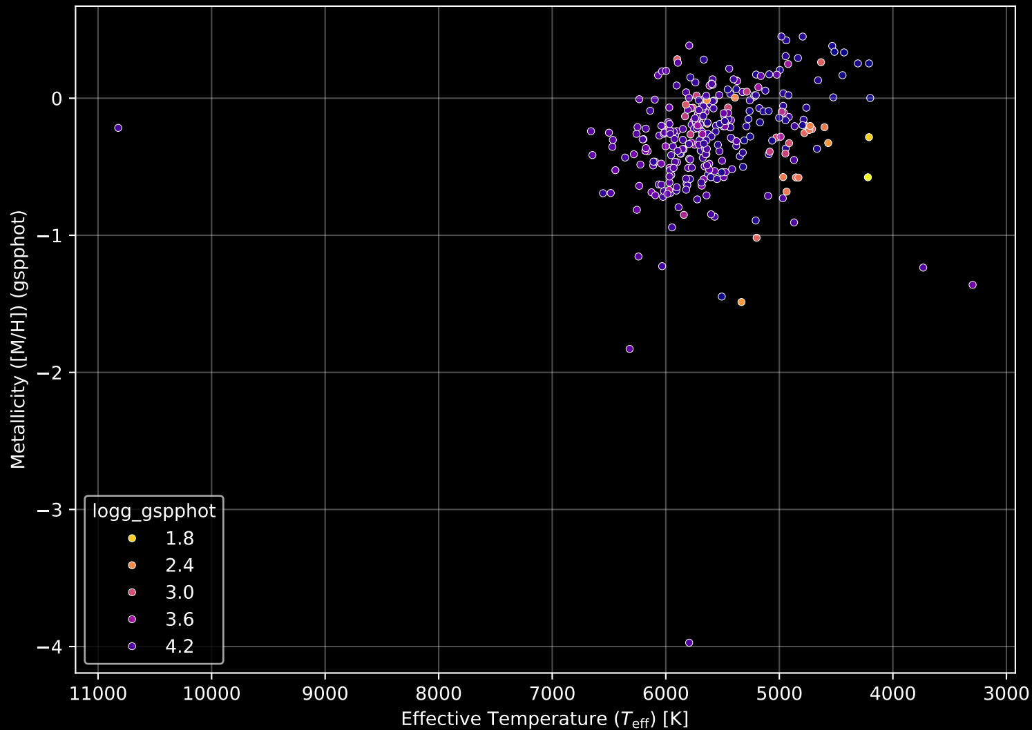
GALAH DR4 Field: [6965] Stellar Population Parameters (n= 306)
